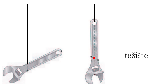
Ilustracija 3.51: Primjer eksperimentalnog određivanja težišta.
