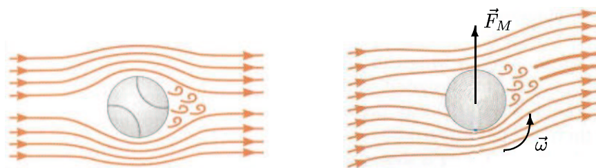
Ilustracija 3.47: Magnusova sila na rotirajuću loptu tijekom gibanja kroz zrak.
