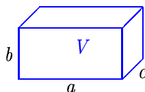
Ilustracija 3.21: Volumen kvadra.
