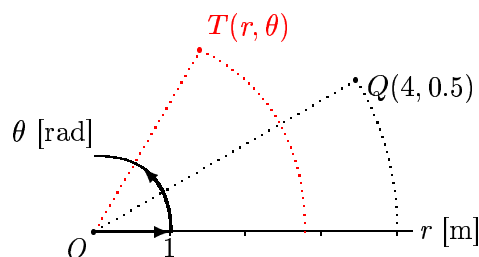
Ilustracija 3.5: Položaj materijalne točke u polarnom koordinatnom sustavu određen je uređenim parom koordinata, (r, \theta) .
