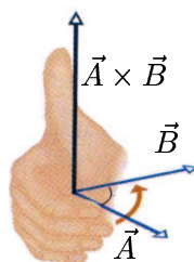
Ilustracija 3.18: Pravilo desne ruke kod određivanja orijentacije vektorskog produkta dvaju vektora.
