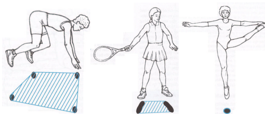
Ilustracija 3.58: Položaji sportaša s različitim stupnjevima stabilnosti.
