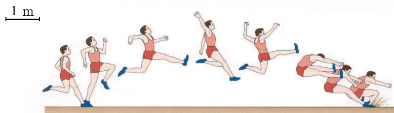
Ilustracija 3.11: Uz određivanje brojčane vrijednosti duljine skoka udalj.
