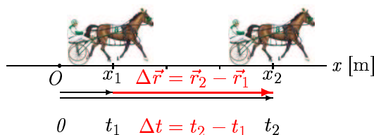
Ilustracija 3.28: Jednoprojektil koji se giba duž osi x od položaja s koordinatom x_1 do x_2 . U trenutku t_1 bio je na mjestu koji je određen položajem \vec{r}_1 , a u trenutku t_2 u položaju \vec{r}_2 .
