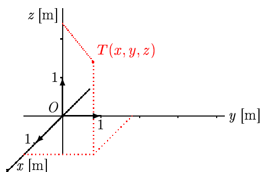
Ilustracija 3.7: Položaj materijalne točke u trodimenzionalnom pravokutnom koordinatnom sustavu određen je uređenom trojkom koordinata, x , y , i z . Na ilustraciji je prikazan desni koordinatni sustav. Lijevi koordinatni sustav dobije se promjenom orijentacije samo jedne koordinatne osi.
