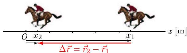
Ilustracija 3.25: Jahač na konju giba se duž osi x od položaja koordinate x_1 = 45 m do položaja x_2 = 5 m.
