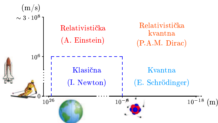
Ilustracija 3.1: Podjela mehanike s obzirom na brzine i dimenzije sustava čija se gibanja izučavaju. Klasičnom se mehanikom mogu izučavati oni sustavi čije su brzine manje od oko 10^6 m/s i dimenzije veće od oko 10^{-8} m.
