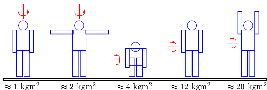
Ilustracija 3.56: Vrijednosti momenta inercije ljudskog tijela.
