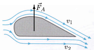
Ilustracija 3.46: Aerodinamička sila na nesimetrično tijelo u gibanju kroz fluid.
