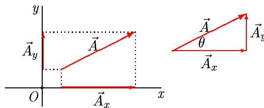
Ilustracija 3.16: Vektorske komponente \vec{A}_x i \vec{A}_y vektora \vec{A} u pravokutnom koordinatnom sustavu.
