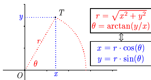
Ilustracija 3.6: Koordinate neke točke u polarnom koordinatnom sustavu, r i \theta , jednoznačno se izražavaju preko koordinata iste točke u pravokutnom koordinatnom sustavu, x i y , i obratno.
