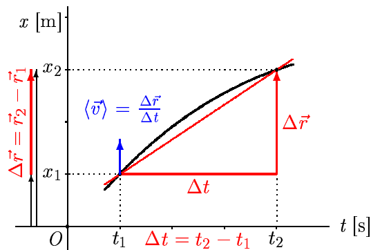
Ilustracija 3.29: Graf položaja materijalne točke u ovisnosti o vremenu. Točke na grafu predstavljaju položaje u odgovarajućim trenucima. Graf se odnosi na jednodimenzionalno gibanje.
