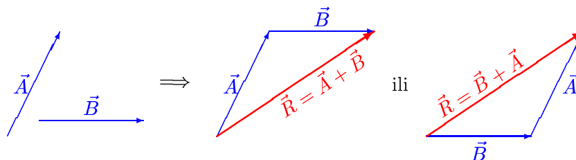
Ilustracija 3.13: Zbrajanje dvaju vektora \vec{A} i \vec{B} , za koje vrijedi zakon komutativnosti.
