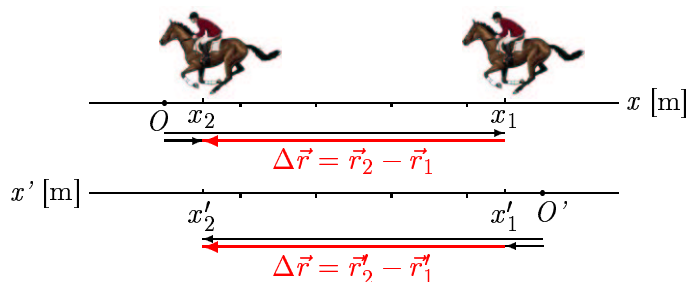
Ilustracija 3.26: Gibanje jahača na konju opisano u dva koordinatna sustava. Pomak jahača ima orijentaciju suprotnu orijentaciji x -osi, ali jednaku orijentaciji x' -osi.
