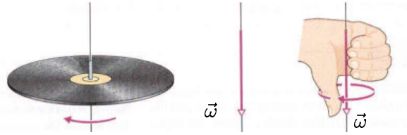
Ilustracija 3.32: Pravilo desne ruke kod određivanja orijentacije vektora kutne brzine. Prsti desne ruke pokazuju rotaciju tijela, a palac orijentaciju vektora kutne brzine \vec{\omega} .
