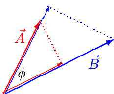
Ilustracija 3.17: Dva vektora \vec{A} i \vec{B} te njihove komponente duž drugog vektora.
