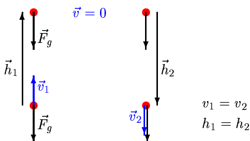
Ilustracija 3.61: Uz određivanje rada sile teže nad tijelom koje je u gibanju uvis i natrag.
