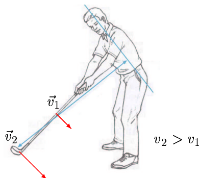
Ilustracija 3.33: Udaljenije točke palice imaju veće iznose tangencijalnih brzina od točaka bližih osi vrtnje.
