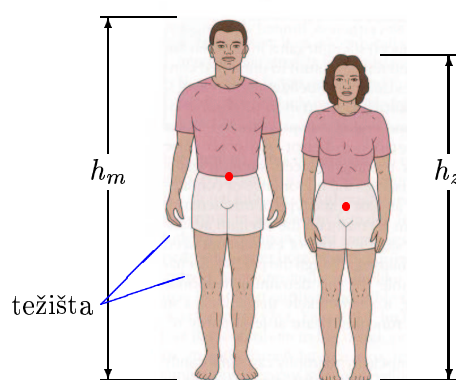
Ilustracija 3.52: U normalnom stojećem položaju, položaj težišta normalnog čovjeka je na 55 do 57 % njegove visine.
